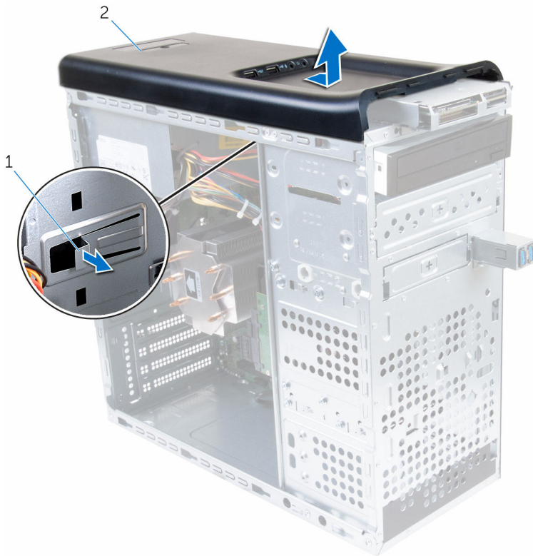
1 Halteklemme
